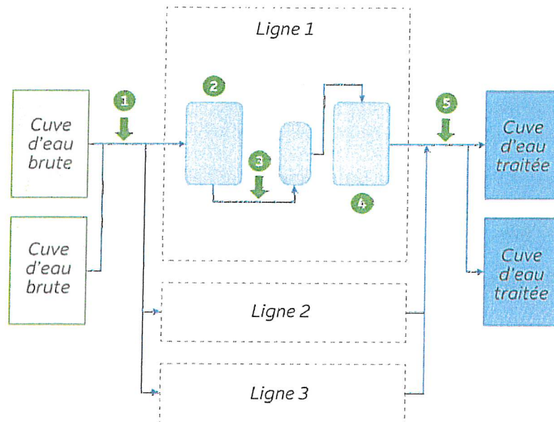
Figure 2 - vue schématique des étapes de traitement
